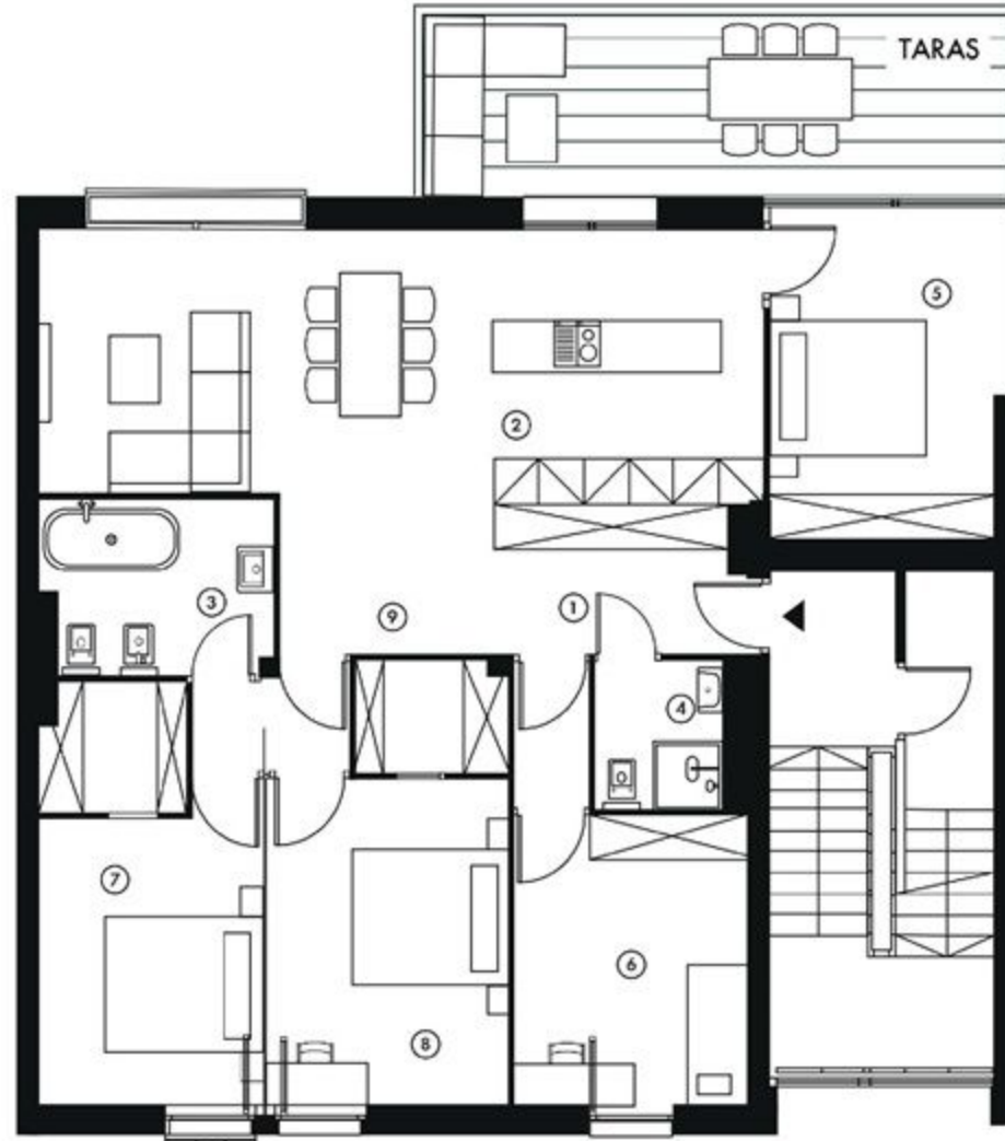
I PIĘTRO (KONCEPCJA)
