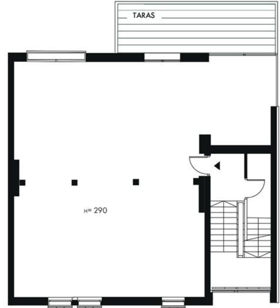
I PIĘTRO (STAN OBECNY)
